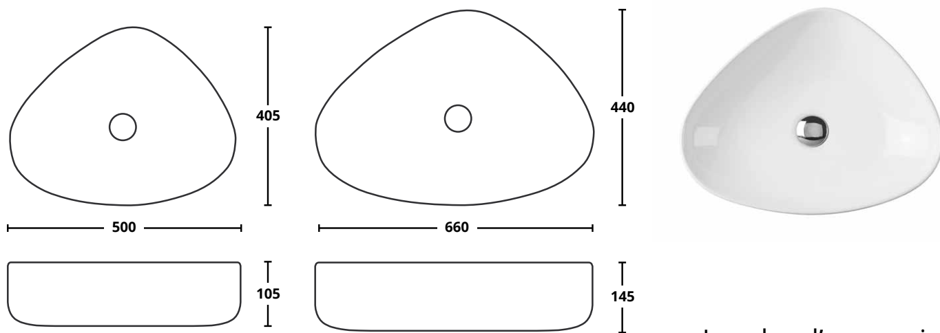
Lavabo d'appoggio Sit on top basin
